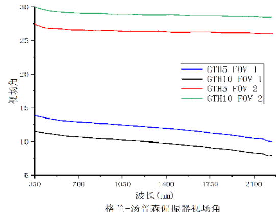
格兰汤姆逊偏振器视场角
