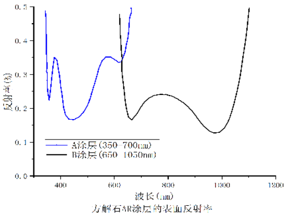
方解石AR涂层的表面反射率
